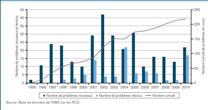
Figure C.4: Problèmes commerciaux spécifiques nouveaux et problèmes commerciaux spécifiques résolus dans le domaine SPS, 1995-2010 (nombre de problèmes)
